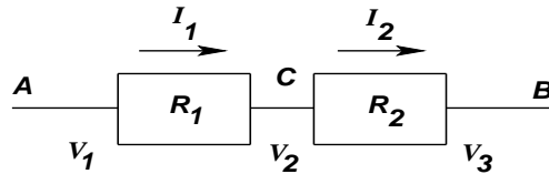
FIG. 2.5 – Résistances en série
