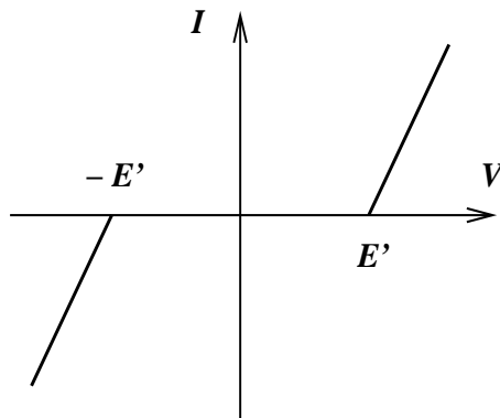
FIG. 2.9 – Caractéristique courant-tension d'un récepteur
