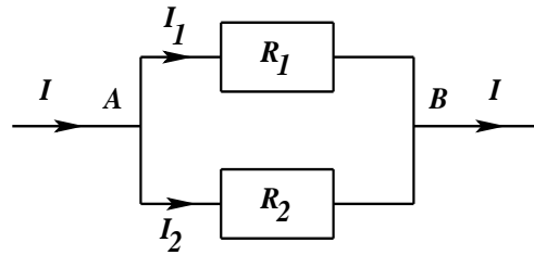
FIG. 2.6 – Résistances en parallèle
