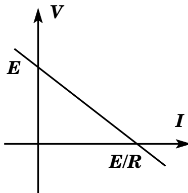
FIG. 2.8 – Caractéristique tension-courant d'un générateur de tension
